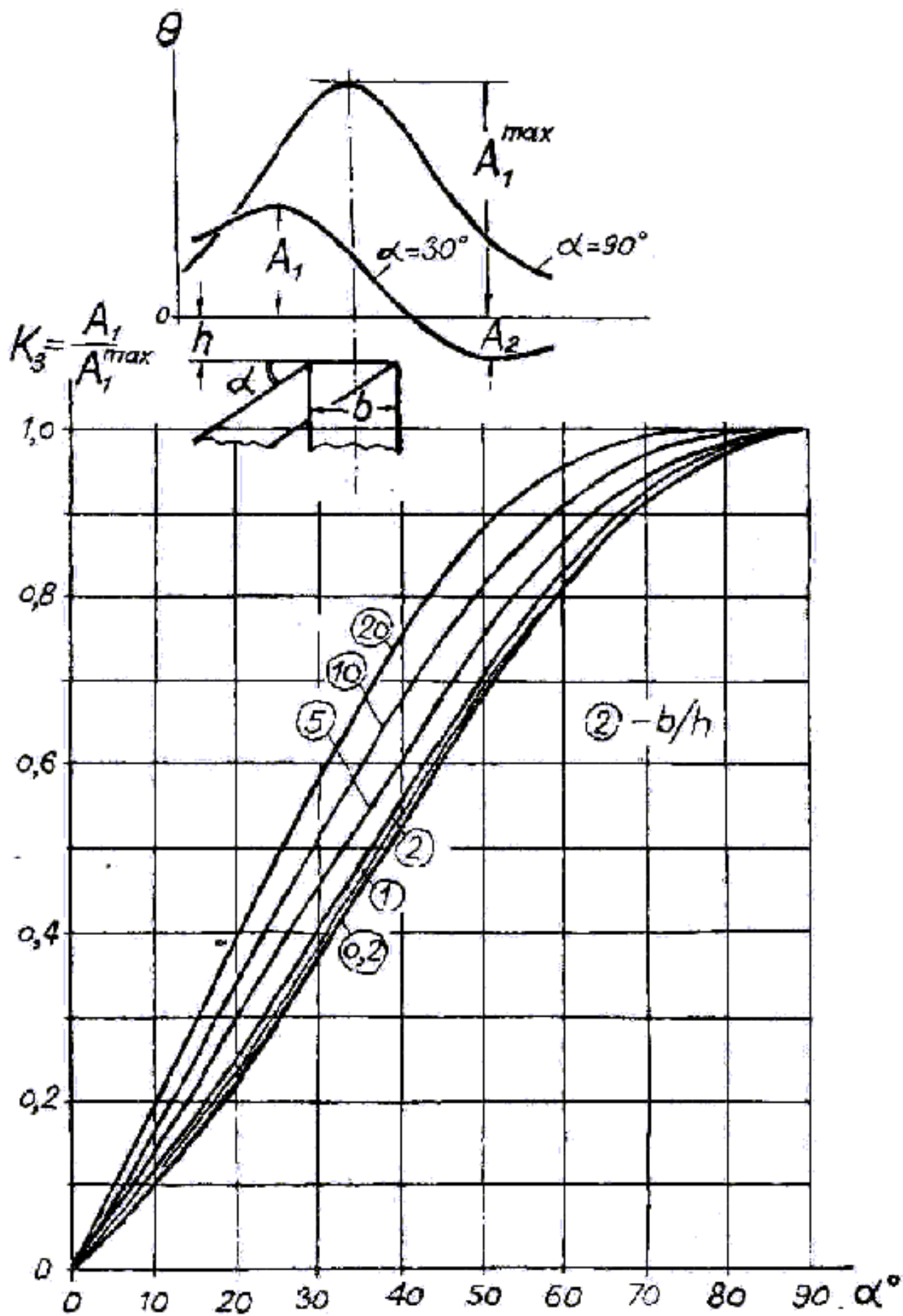
Рис. 1.11 Номограмма зависимости K_3 = A_1/A_1^{max} от угла \alpha .
