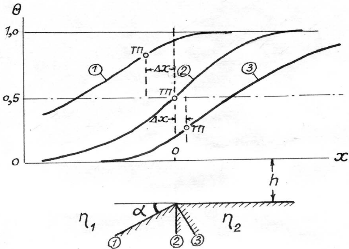
Рис.2.2. График \theta над наклонным уступом 1- \alpha < 90^\circ ; 2- \alpha = 90^\circ ; 3- \alpha > 90^\circ .
