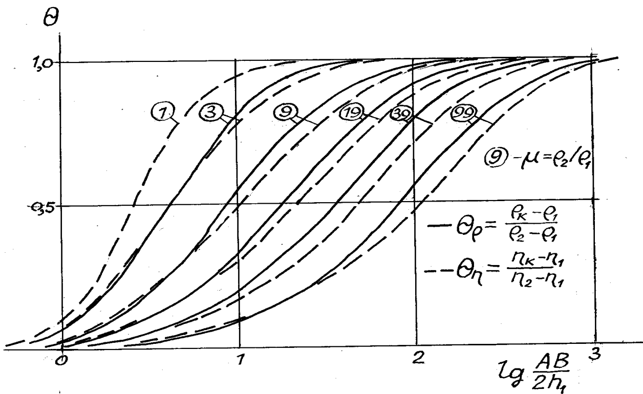
Рис. 3.3. К выбору разносов установки в двухслойной среде по нормированному аномальному параметру \theta ( \rho_1, \eta_1, h_1 – параметры верхнего слоя, \rho_2, \eta_2 – параметры подстилающей среды).
