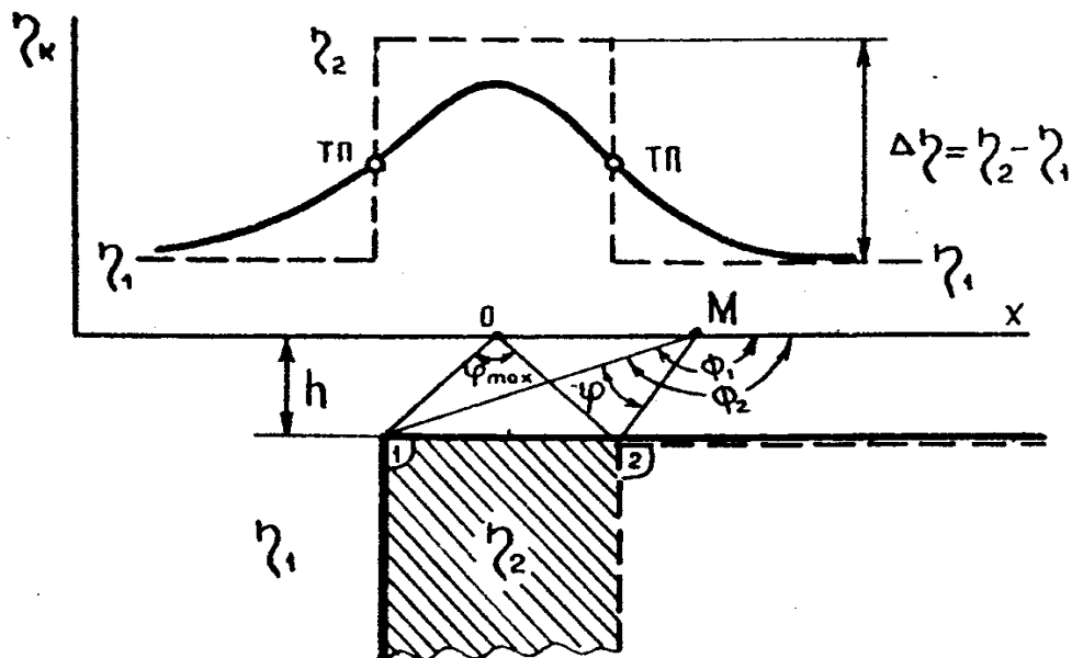
Рис. 1.3. График \eta_k над вертикальным пластом. ТП – точки перегиба графика.
