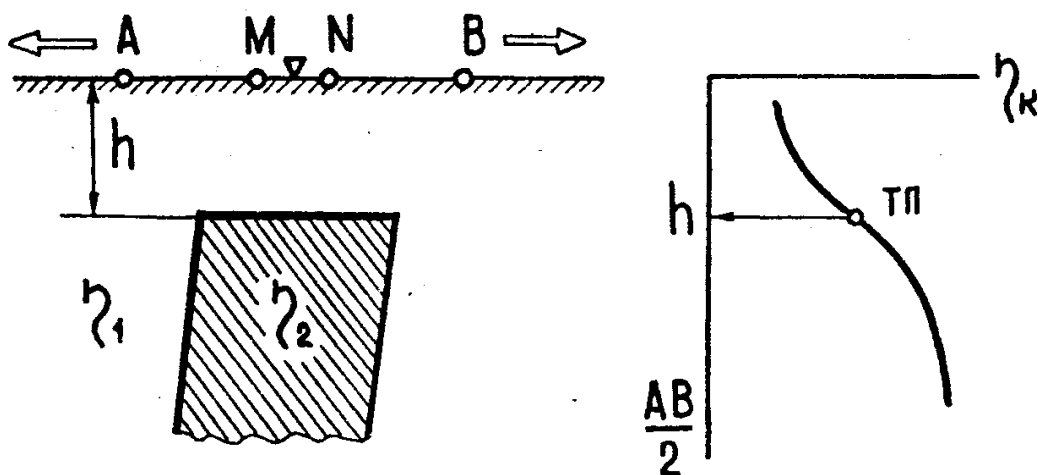
Рис. 1.6. К оценке залегания верхней кромки пласта по данным ВП–ВЭЗ.
