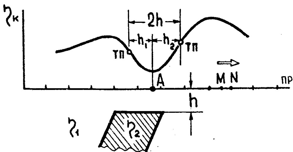
Рис. 1.7. К оценке глубины залегания верхней кромки пласта по данным ВП–СГ.
