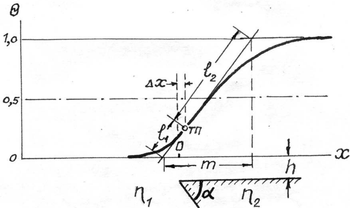
Рис. 2.3 К оценке элементов залегания наклонного уступа.
