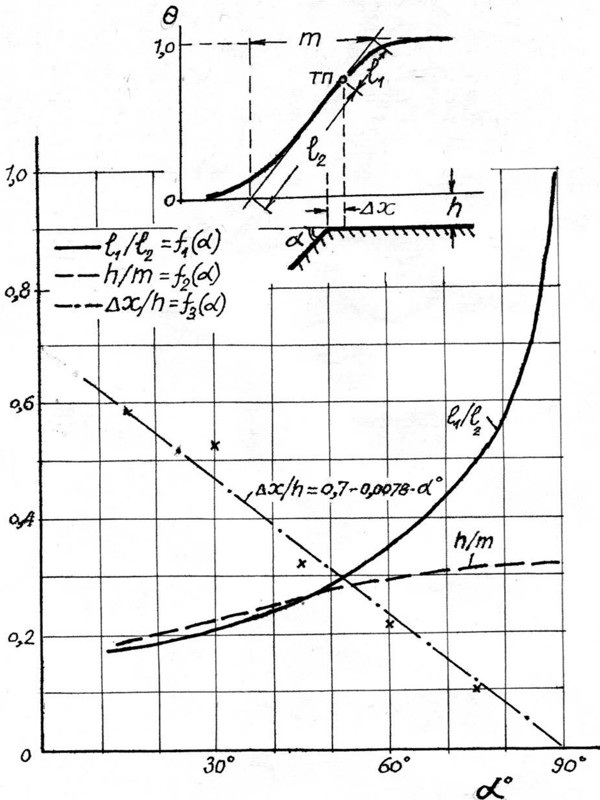
Рис. 2.4. Номограмма для оценки элементов залегания наклонного уступа l_1/l_2, h/m, \Delta x/h от угла \alpha .
