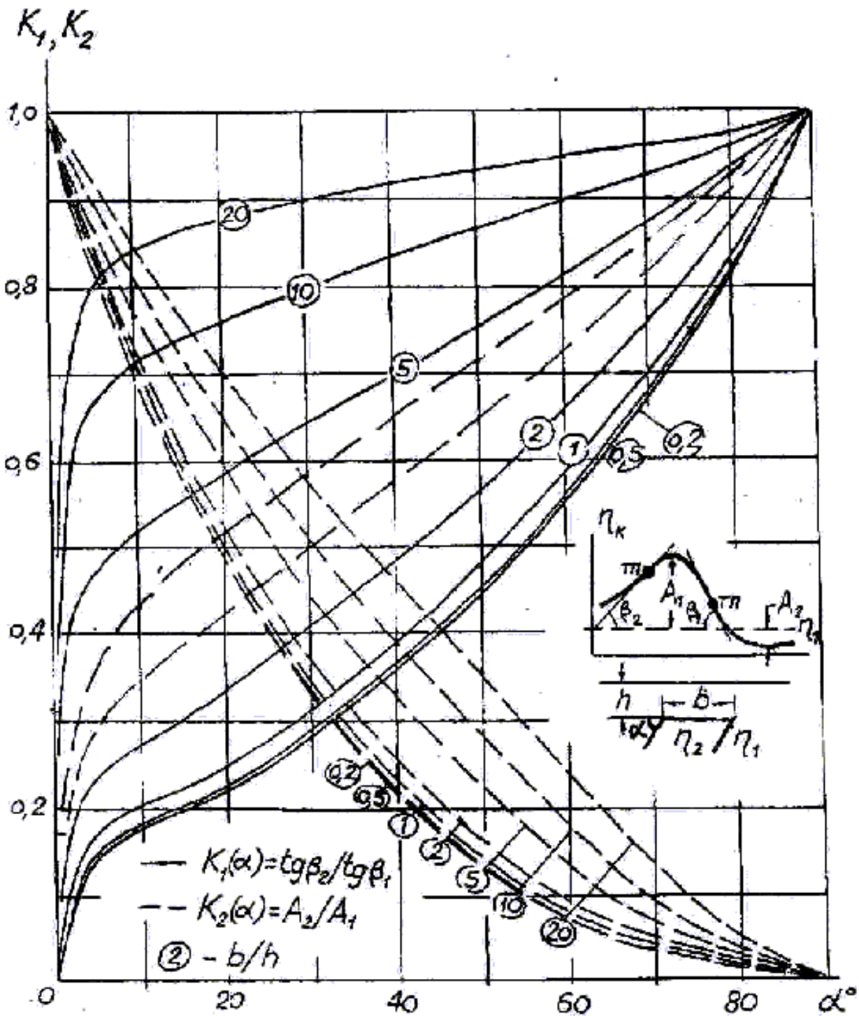
Рис. 1.10. Номограмма зависимостей K_1(\alpha) = \text{tg} \beta_2 / \text{tg} \beta_1 и K_2(\alpha) = A_2 / A_1 .
