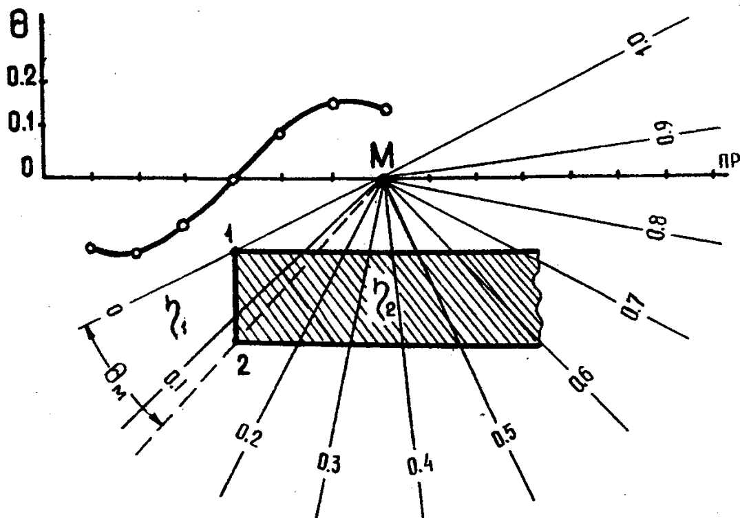
Рис. 1.5. К расчету поля \eta_k по углу видимости.
