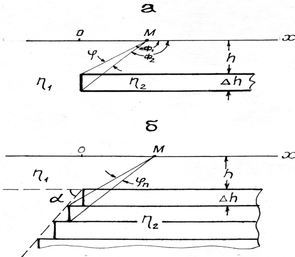
Рис.2.1. К расчёту поля \eta_k наклонного уступа : а – для горизонтальной полупластины; б – для наклонного уступа;
