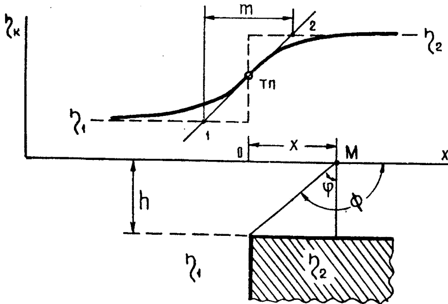
Рис. 1.2. График \eta_k над вертикальным уступом.
