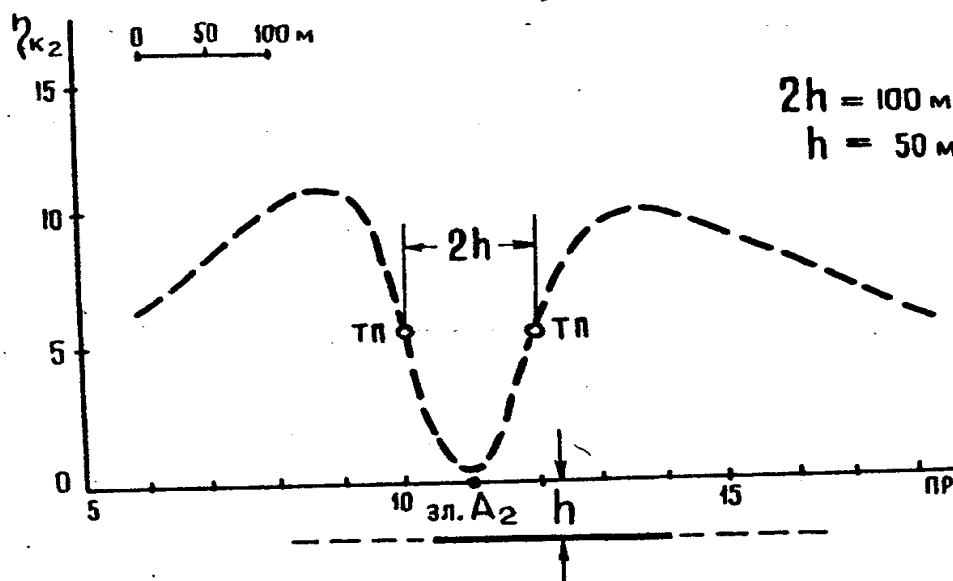
Рис. 3.2. К оценке глубины до верхней кромки пласта
