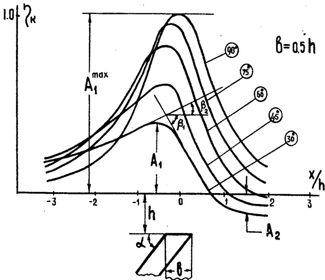
Рис. 1.8. Графики \eta_k для наклонного пласта.
